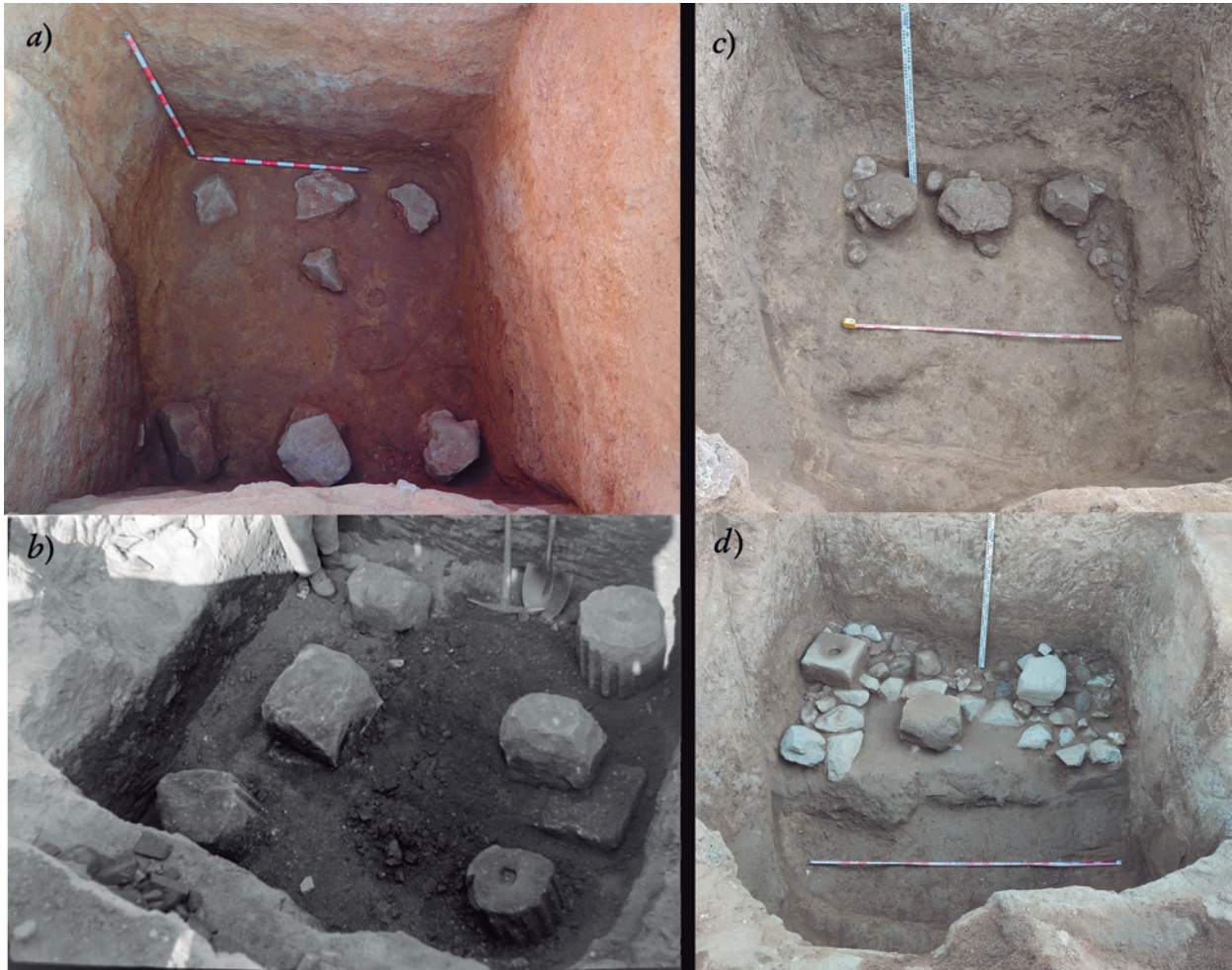
FIGURA 21. Fosses de maniobra de l'Estrella (fossa 1 i 2) i Can Peixau: a) la fossa 1, b) la fossa de Can Peixau, c) la fossa 2 i d) la fossa 2 modificada. Font: Iñaki Moreno i Josep Cortinas, Arxiu J. M. Cuyàs.
